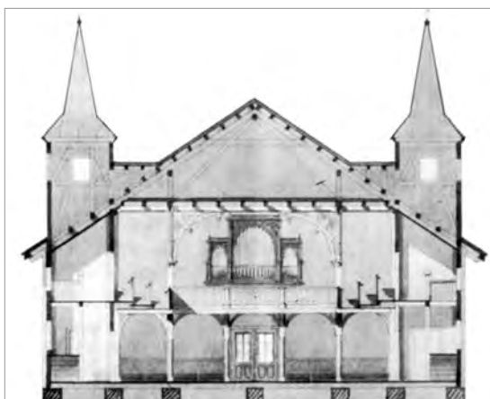
Tversnitt av kirken med orgelet. Etter originaltegningene.
