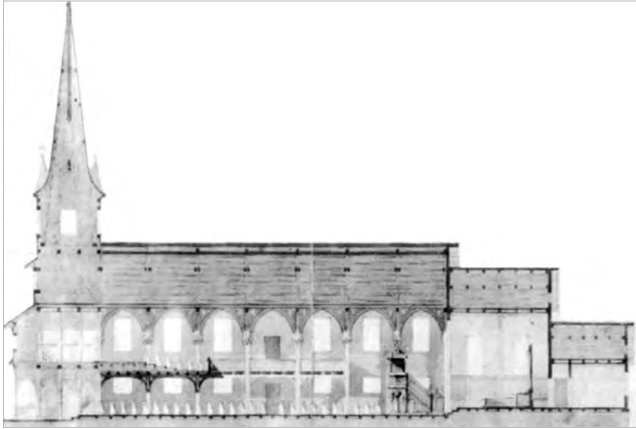
Skåtøy kirke, langsnitt etter originaltegningene av arkitektene Schirmer og von Hanno.
