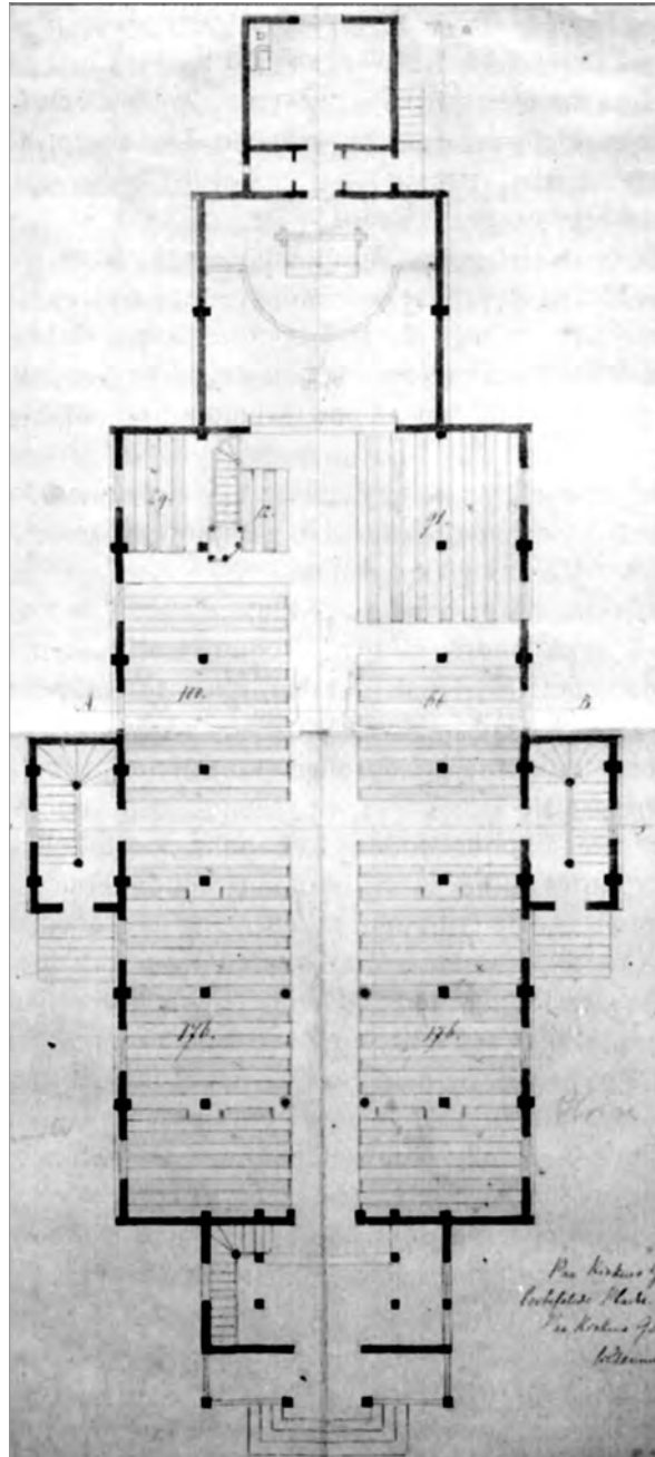
Grunnplan av kirkens gulv. Arkitektene regnet med at det på kirkens gulv var plass til 645 personer, mens galleriet kunne romme 255, tilsammen 900 mennesker. Originaltegning av Schirmer og von Hanno.
